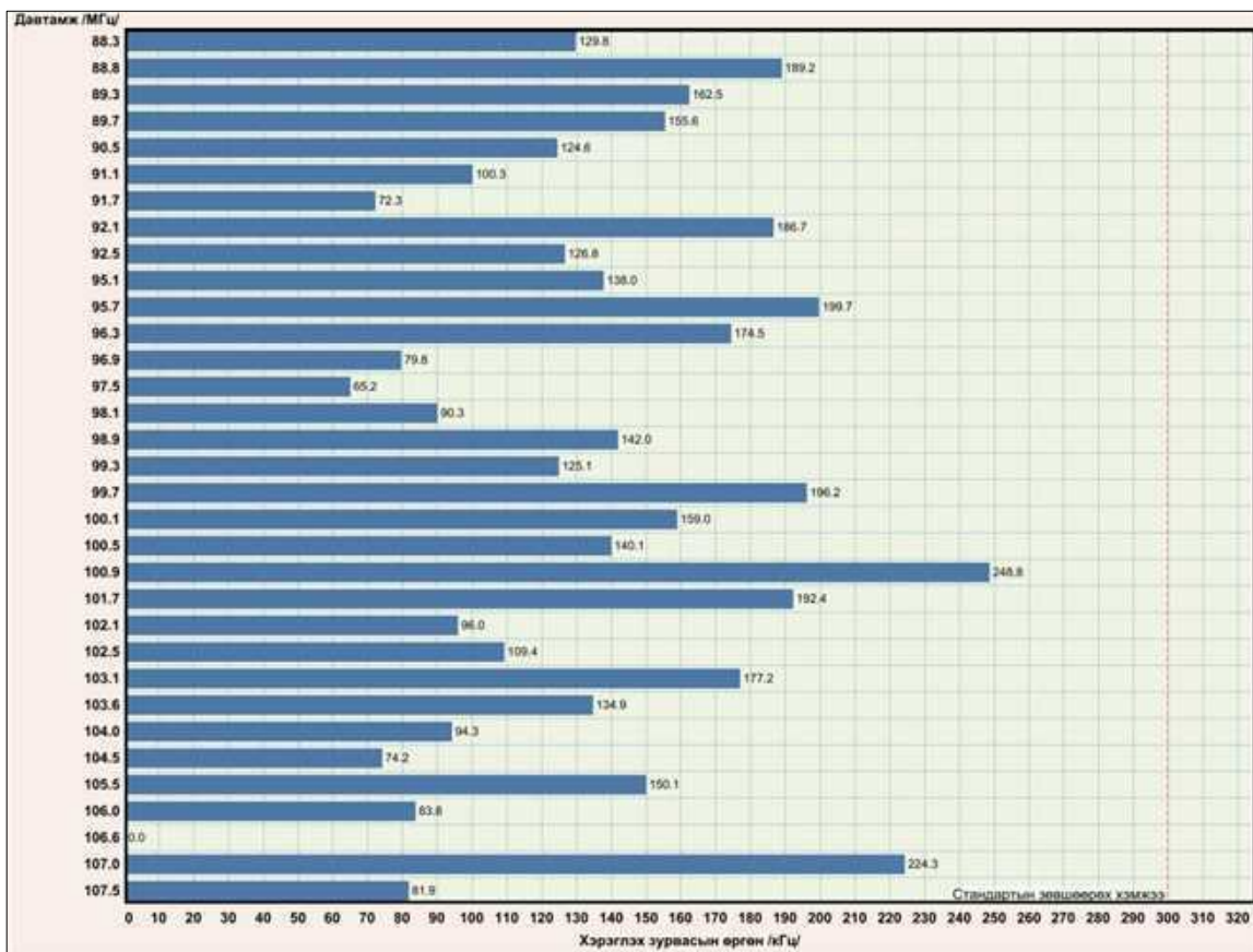
Зураг 4. Хэрэглэх зурвасын өргөний хэмжилтийн үр дүн.
