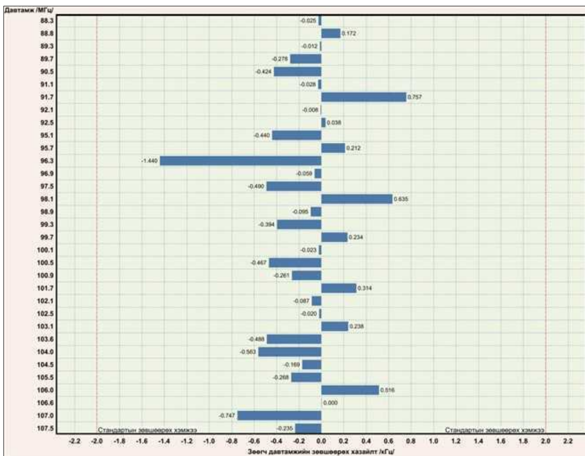
Зураг 5. Зөөгч давтамжийн зөвшөөрөх хазайлтын хэмжилтийн үр дүн.
