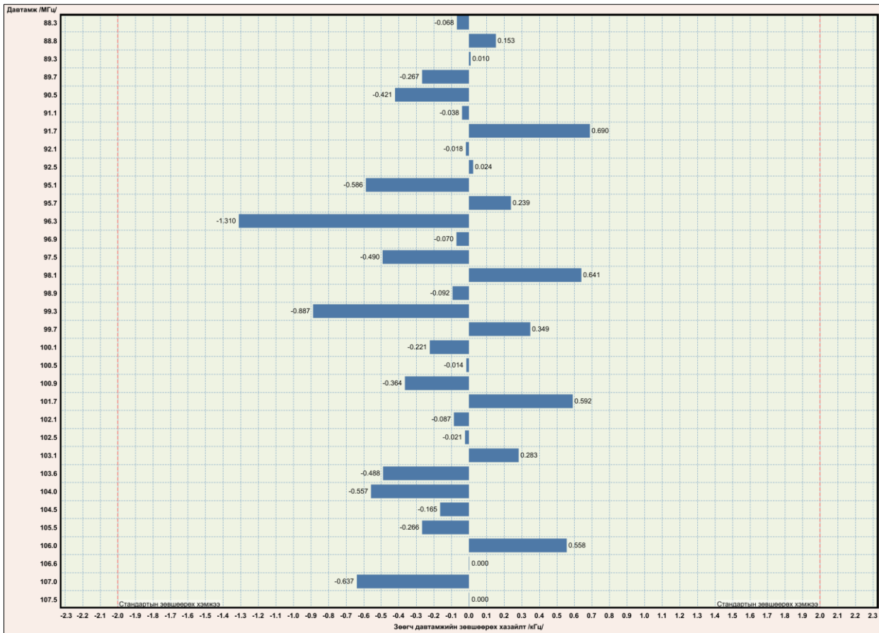
Зураг 5. Зөвч давтамжийн зөвшөөрөх хазайлтын хэмжилтийн үр дүн
