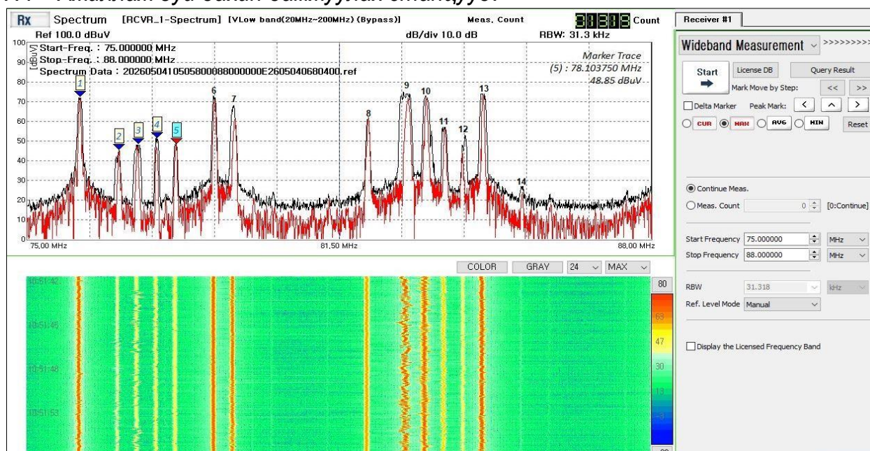
Зураг 7. Радио давтамжийн 75-88 МГц-ийн зурвасын хэмжилт
