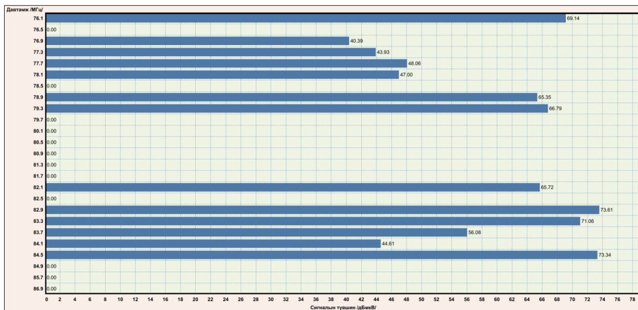
Зураг 8. Радио давтамжийн 75-88 МГц-ийн зурваст хэмжигдсэн дохионы түвшин.
