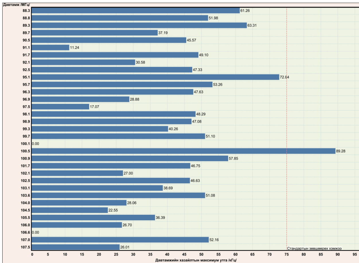
Зураг 7. Давтамжийн хазайлтын максимум утгын хэмжилтийн үр дүн
