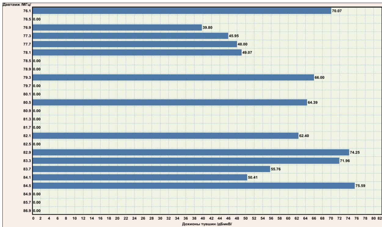
Зураг 9. Радио давтамжийн 75-88 МГц-ийн зурваст хэмжигдсэн дохионы түвшин.
