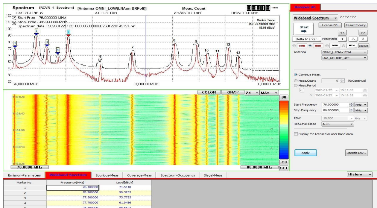
Зураг 8. Радио давтамжийн 75-88 МГц-ийн зурвасын хэмжилт
