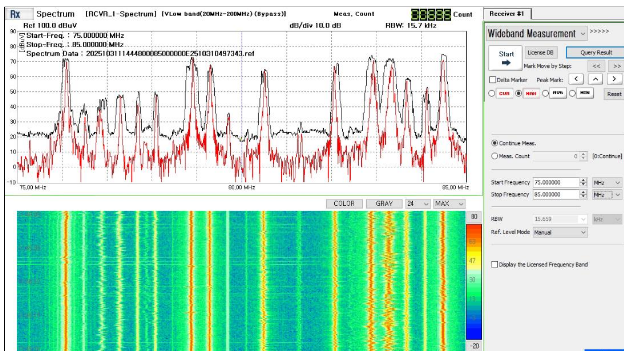
Зураг 7. Радио давтамжийн 75-85 МГц-ийн зурвасын хэмжилт
