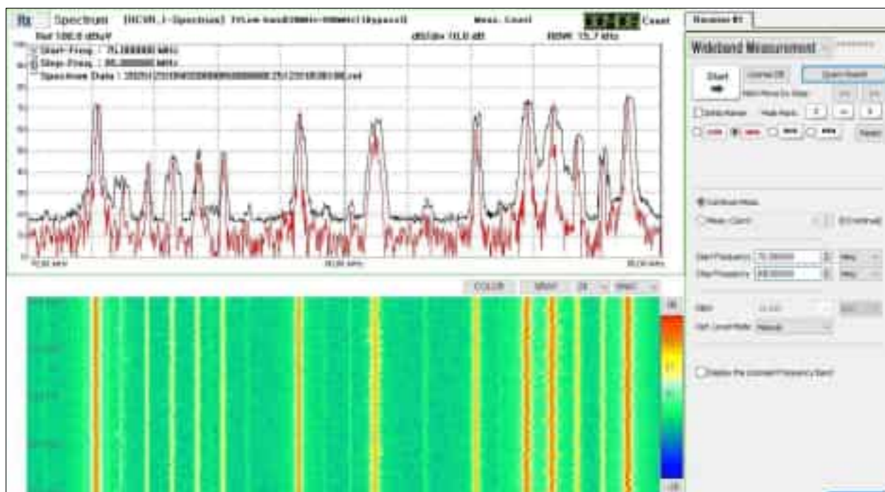
Зураг 7. Радио давтамжийн 75-85 МГц-ийн зурвасын хэмжилт
