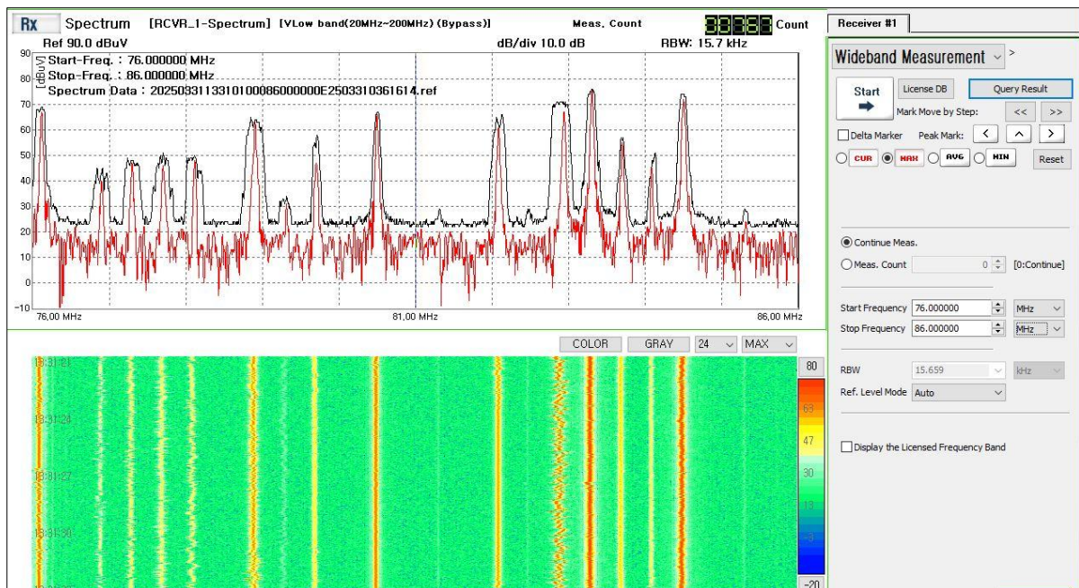
Зураг 7. Радио давтамжийн 76 МГц-86 МГц-ийн зурвасын хэмжилт
