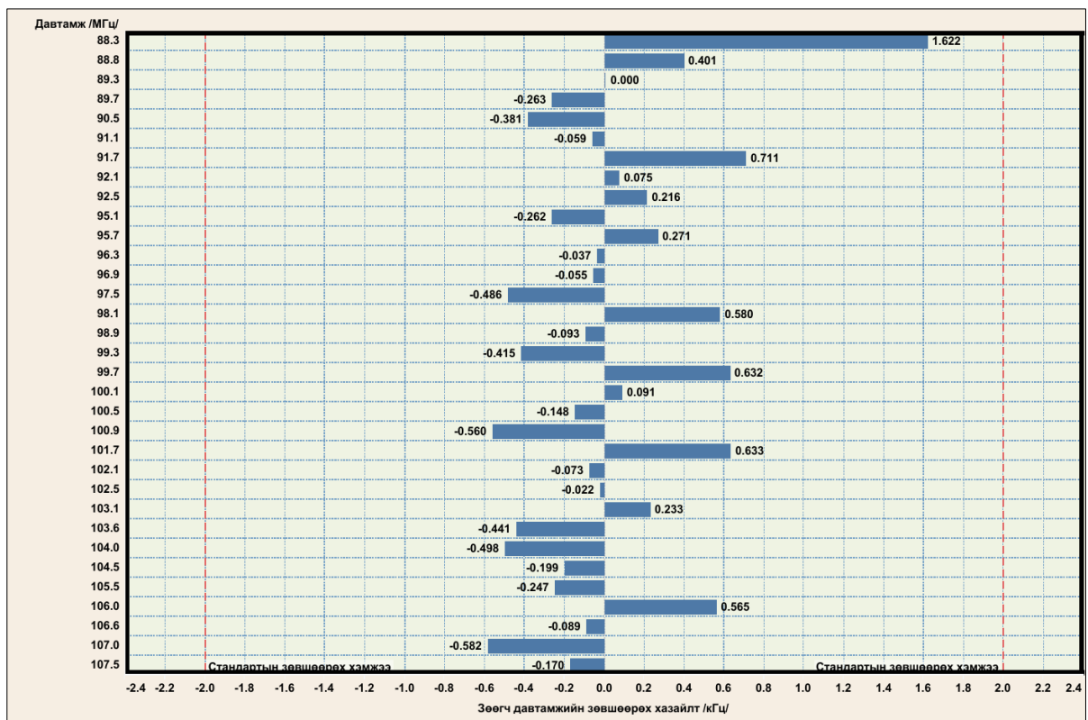
Зураг 4. Зөөгч давтамжийн зөвшөөрөх хазайлтын хэмжилтийн үр дүн
