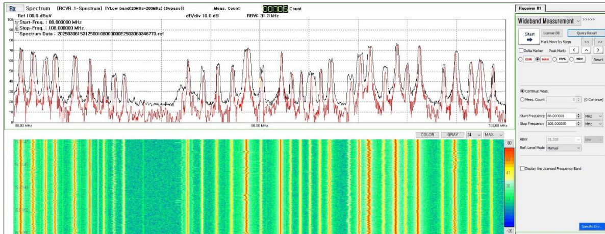
Зураг 2. Радио давтамжийн 88-108 МГц-ийн зурвасын хэмжилт
