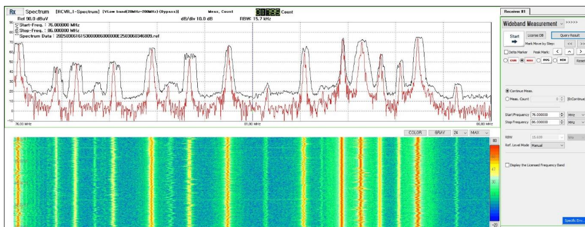
Зураг 7. Радио давтамжийн 76 МГц-86 МГц-ийн зурвасын хэмжилт
