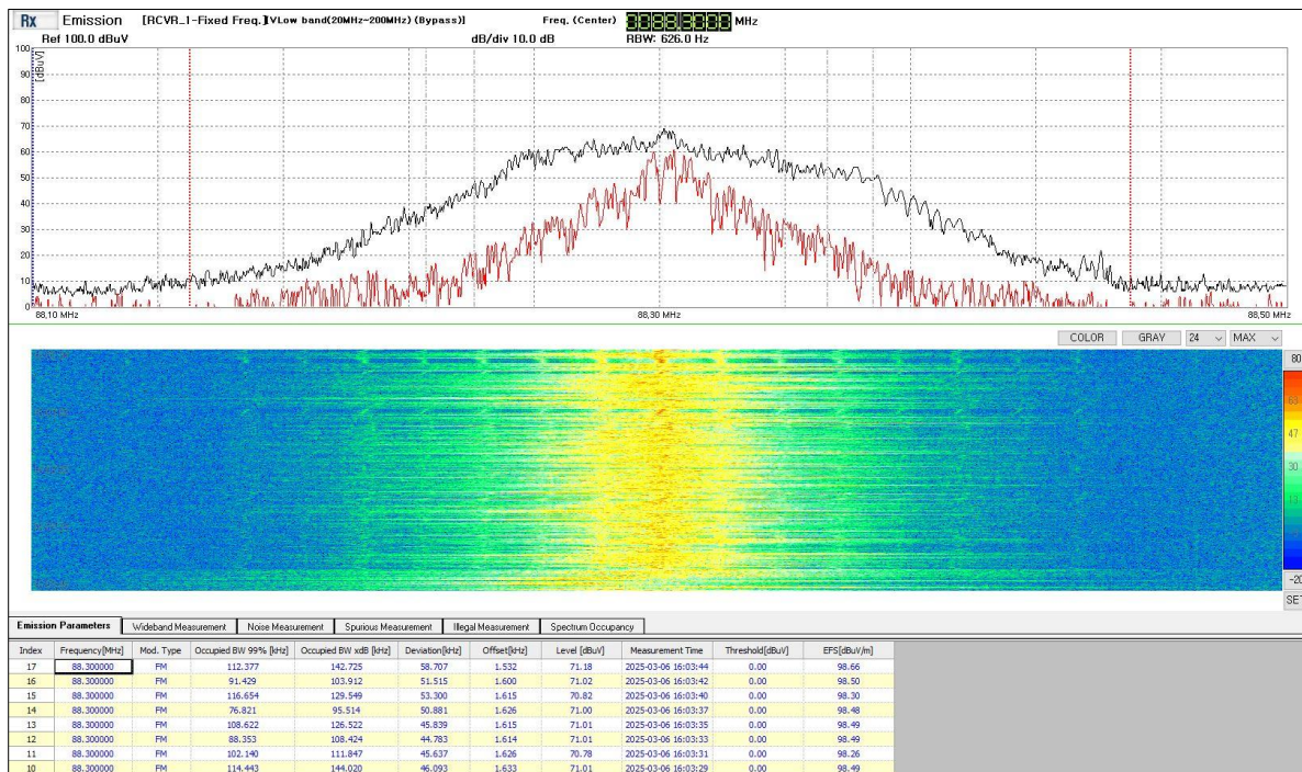
Зураг 3. Радио давтамжийн 88-108 МГц-ийн зурвасын хэмжилт
