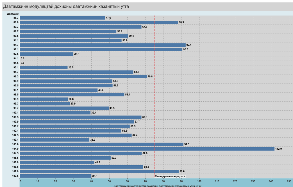
Зураг 2. Давтамжийн модуляцтай дохионы давтамжийн хазайлтын утга
