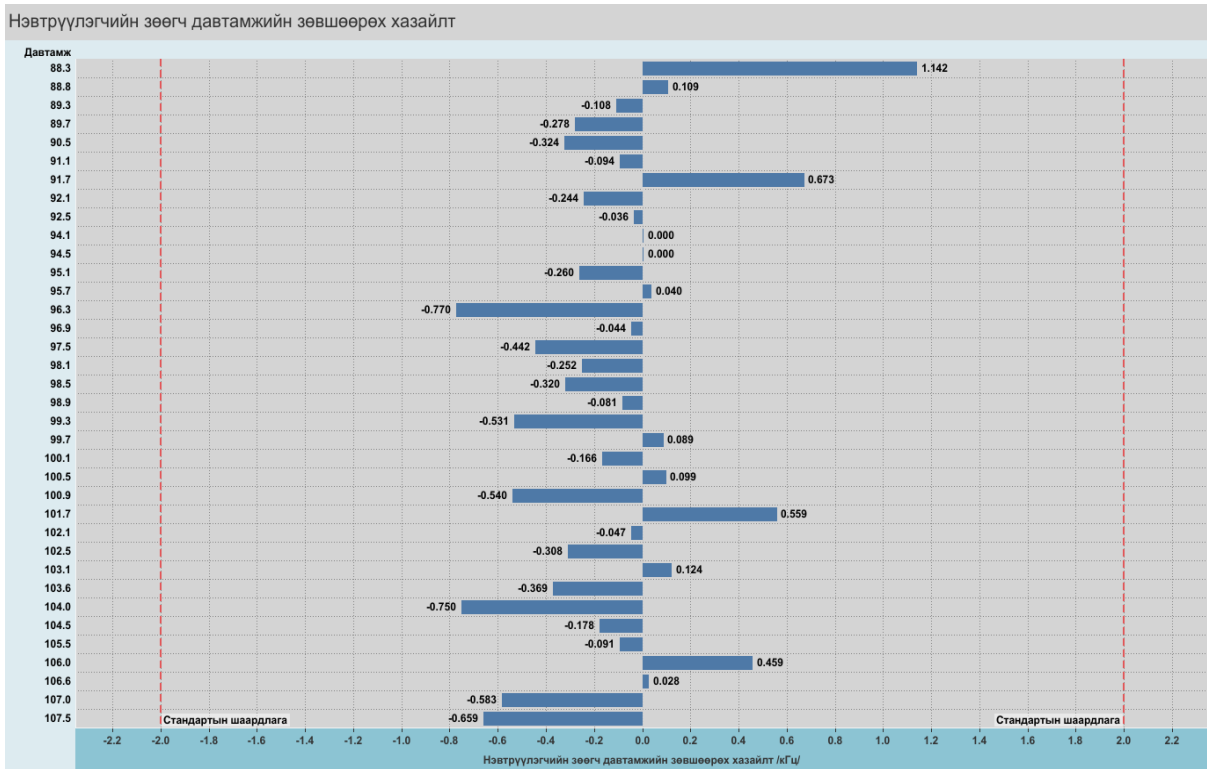
Зураг 3. Нэвтрүүлэгчийн зөөгч давтамжийн зөвшөөрөх хазайлт
