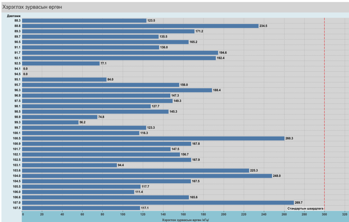
Зураг 4. Хэрэглэх зурвасын өргөн
