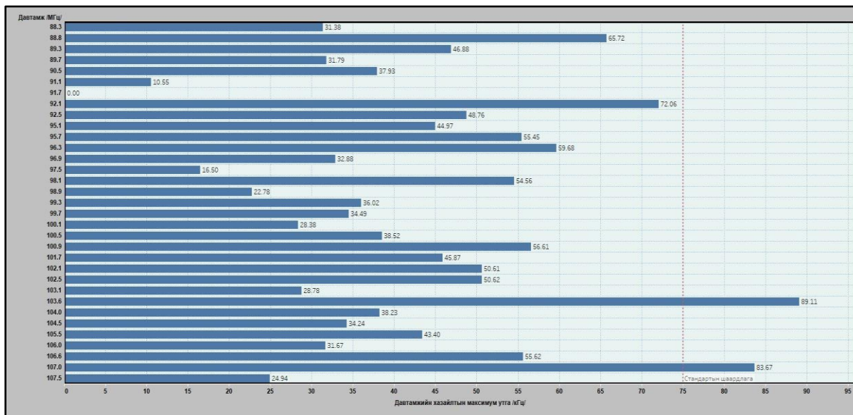
Зураг 6. Давтамжийн хазайлтын максимум утгын хэмжилтийн үр дүн
