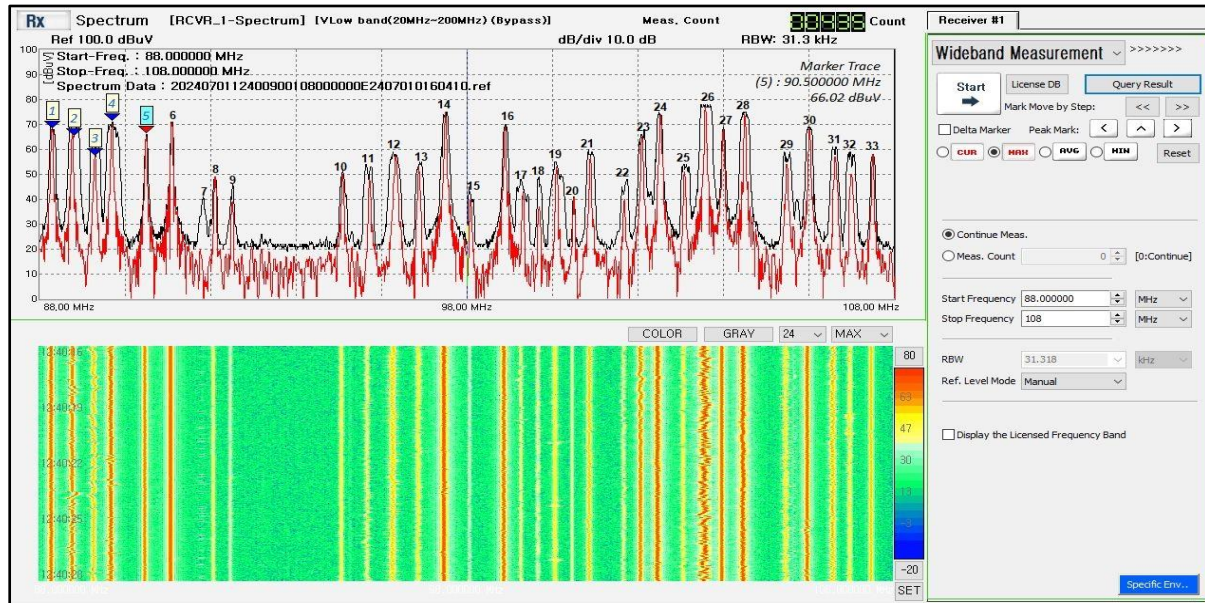
Зураг 2. Радио давтамжийн 88 МГц-108 МГц-ийн зурвасын хэмжилт
