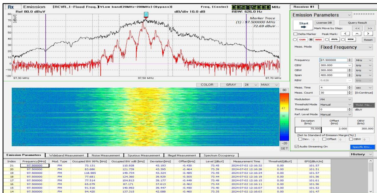
Зураг 3. FM радиогийн нэвтрүүлэх станцын дохионы параметруудийг хэмжиж байгаа нь
