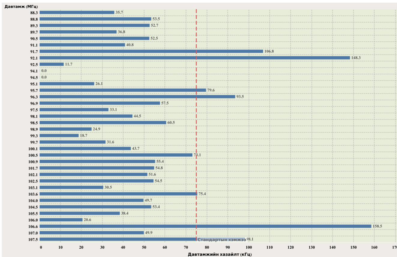
Зураг 3. Давтамжийн хазайлт.
