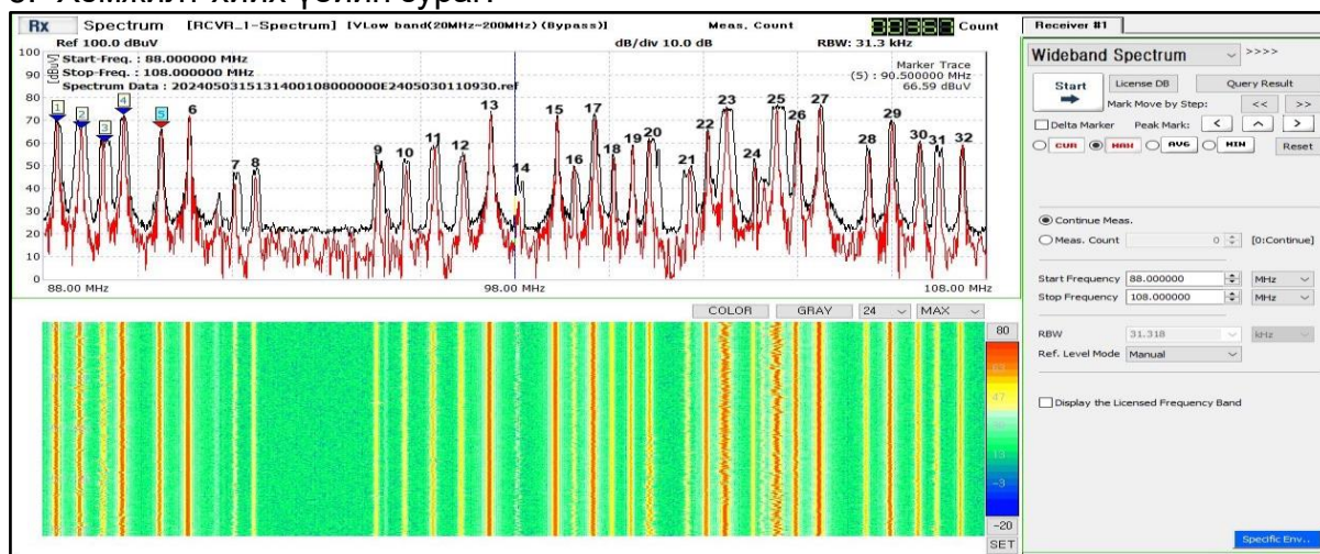
Зураг 3. Радио давтамжийн 88 МГц-108.0 МГц-ийн зурвасын хэмжилт
