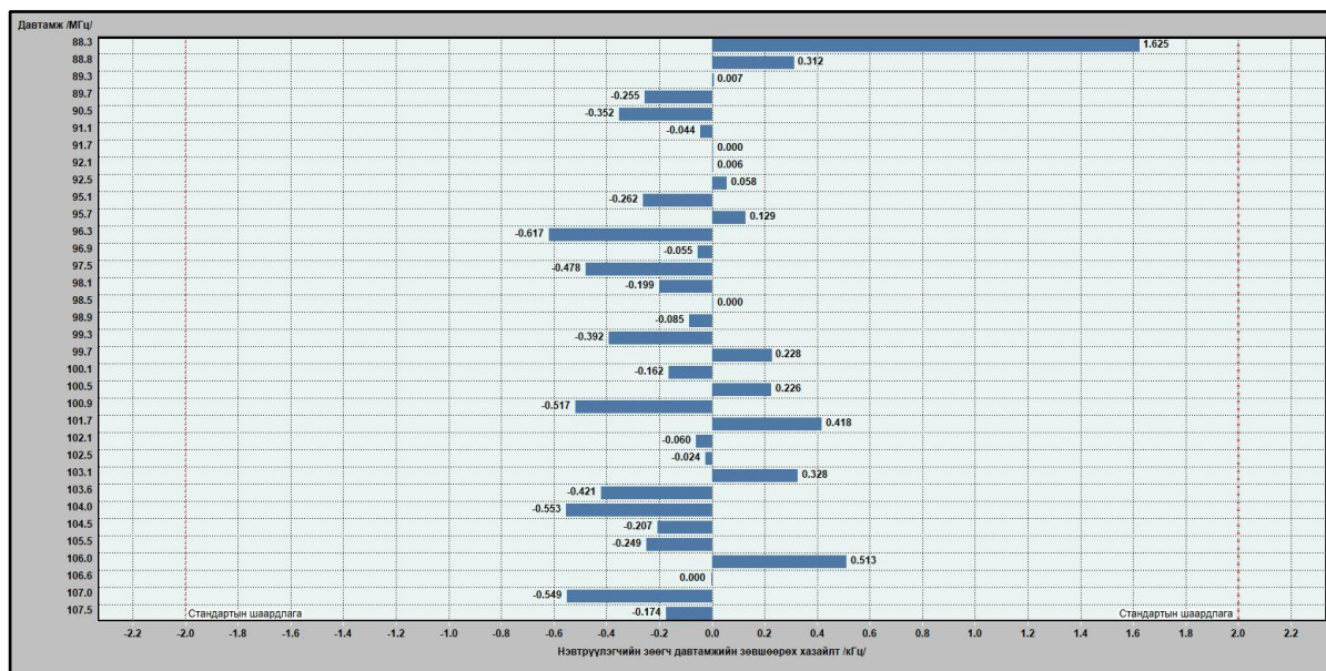
Зураг 4. Зөөгч давтамжийн зөвшөөрөх хазайлтын хэмжилтийн үр дүн
