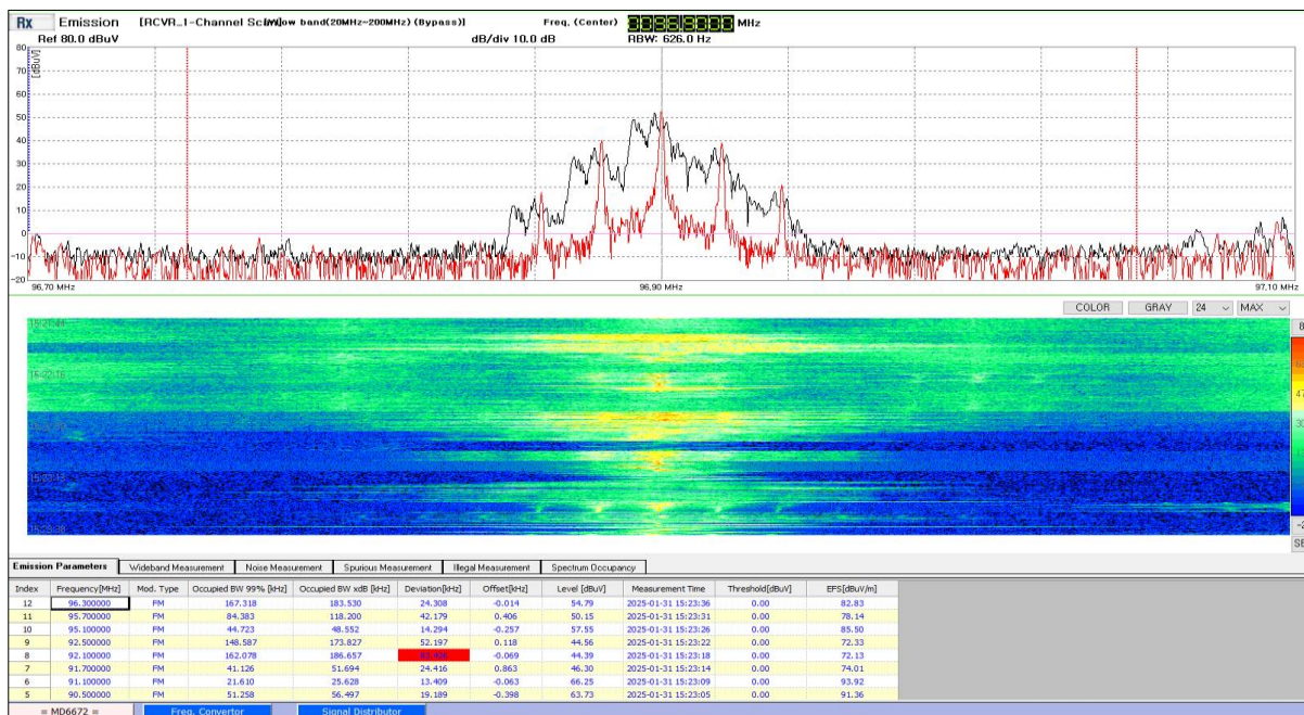
Зураг 3. Радио давтамжийн 88-108 МГц-ийн зурвасын хэмжилт
