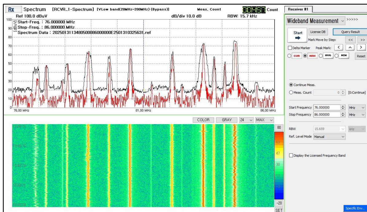
Зураг 7. Радио давтамжийн 76 МГц-86 МГц-ийн зурвасын хэмжилт
